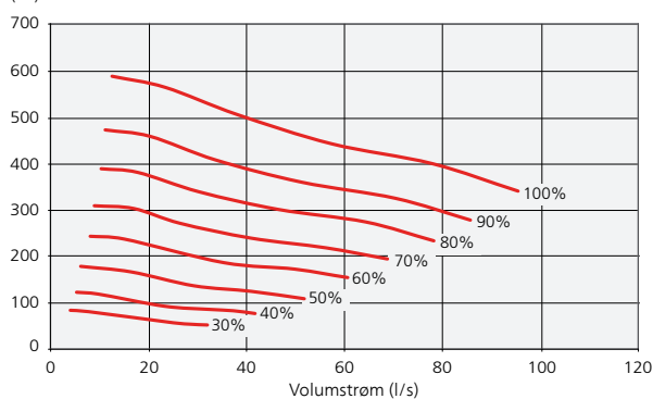
Effekt likestrømvifte
