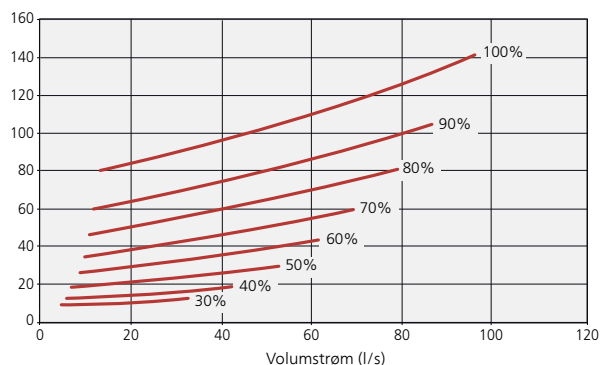
Effekt likestrømvifte
